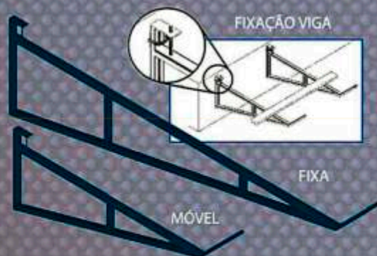
FIXA - 2,50 X 0,80M MÓVEL - 1,40 X 0,80M
