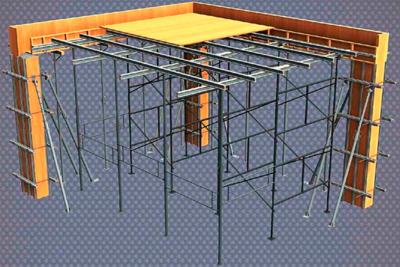
SISTEMA DE ESCORAMENTO
